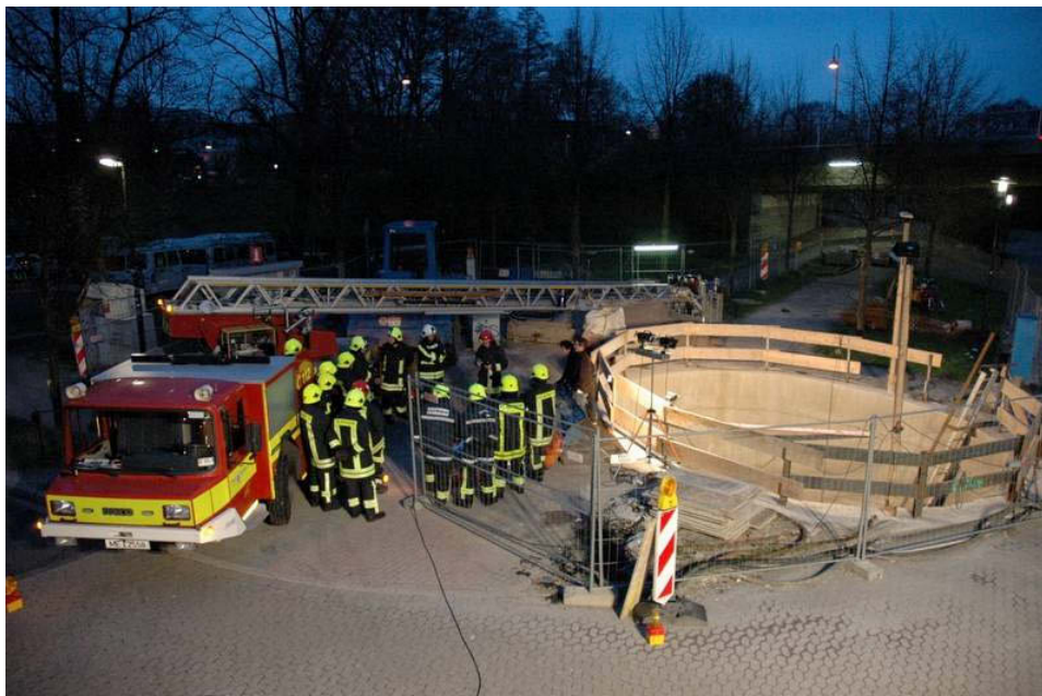
Rettung über die Drehleiter aus einer Startgrube der Überdruckbaustelle
