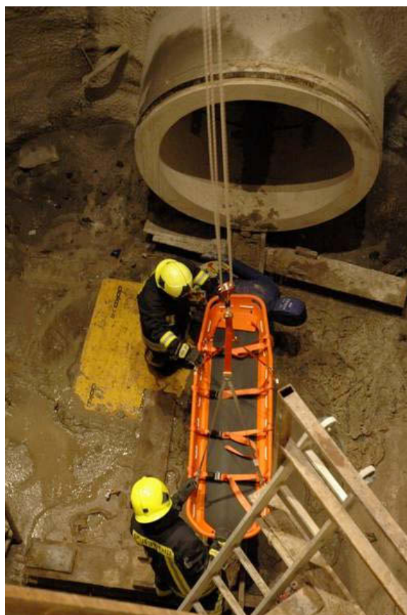
Rettung über die Drehleiter aus einer Startgrube der Überdruckbaustelle
